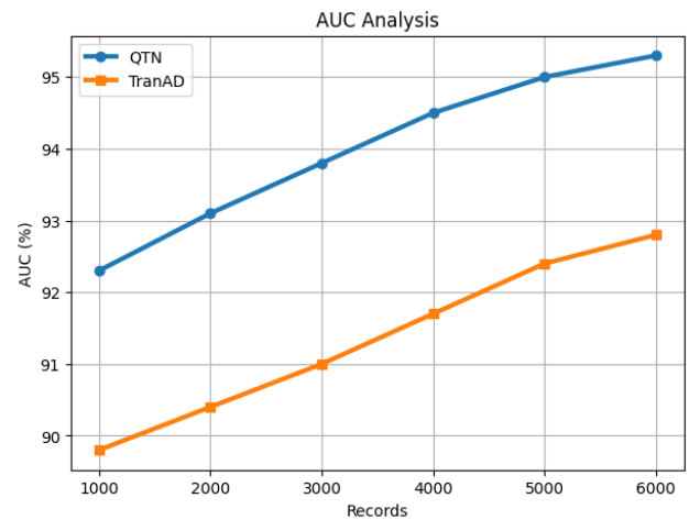
Fig 8: AUC Analysis
